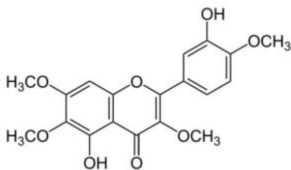
קסטיצין - מבנה המולקולה
