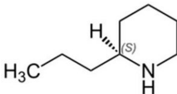
מבנה מולקולת הקונין
