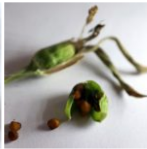
אגרוסטמת השדות. צילמה: ערגה אלוני © מימין לשמאל לפי הסדר - ההלקט מוגן בגביע; הלקט סגור והלקט פתוח ובו זרעים בשלים; פני הזרע מכוסים גבשושיות; זרעים לא-אחידים בצורה ובגודל להגדלה - לחצו על התמונות
