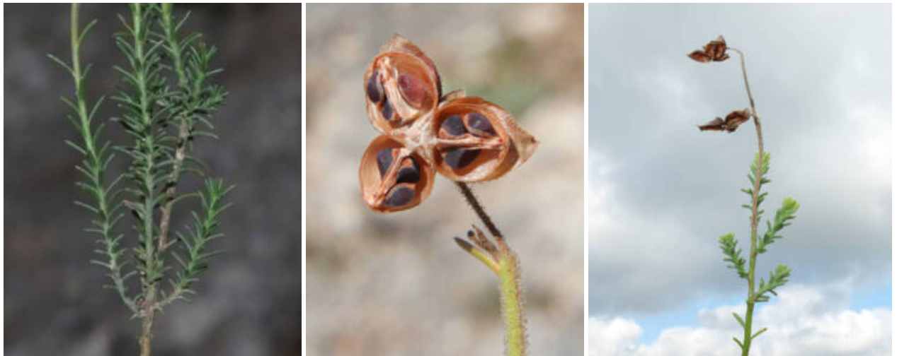
מימין ואמצע: לוטמית המטאטא Fumana scoparia , צילם עוז גולן © , משמאל: לוטמית המטאטא Fumana scoparia , צילם נוגן צברי ©
